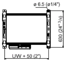
Рис. 2-5б Диаграмма отверстий для монтажа к полу (UW=720/760/820 мм).
