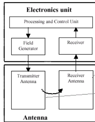
Рис. 1-1 Блок-схема металлодетектора
