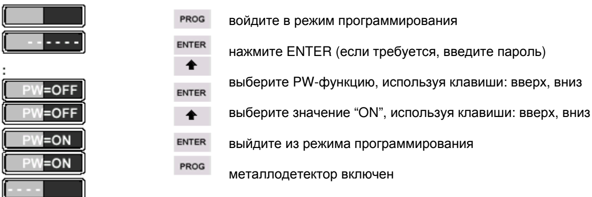
Рис. 21b Включение металлодетектора
