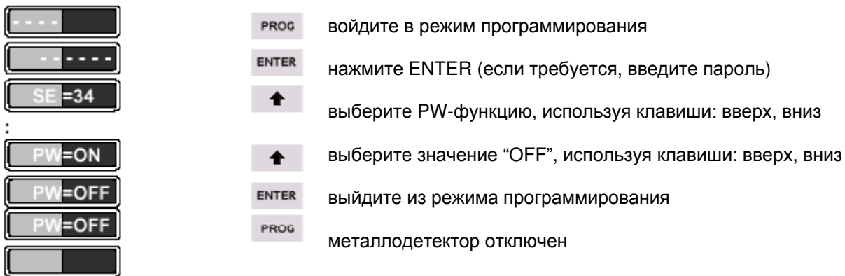
Рис. 21а Отключение металлодетектора
