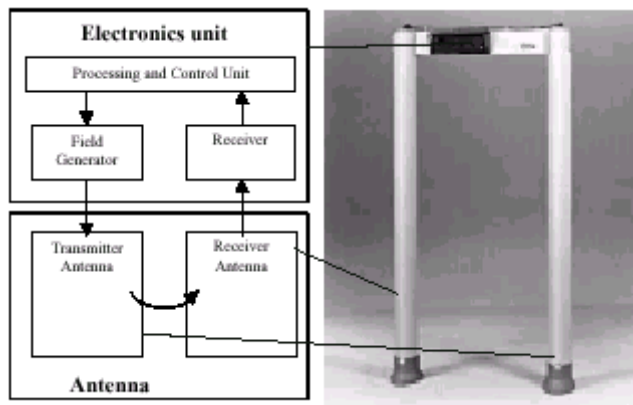
Рис. 1 Блок-схема металлодетектора
