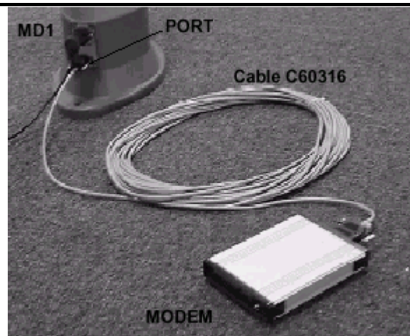
Рис. 26 Подключение металлодетектора к модему
