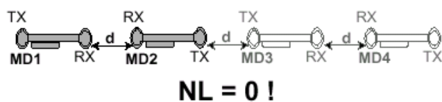
Рис. 11 Установка 3 или 4 металлодетекторов ( d \geq 30 см).
