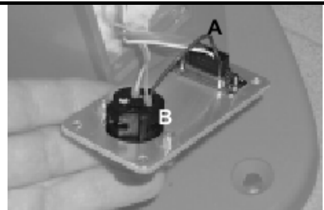
Рис. 31d – вставьте синий провод в соединительное гнездо источника питания (другой конец синего провода уже подключен)
