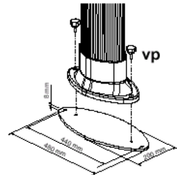
Рис. 13 Расположение отверстий для монтажа дополнительных металлических пластин
