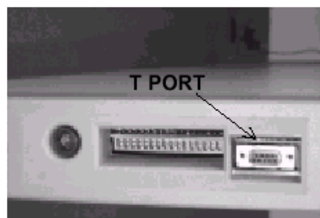
Рис. 4-5 Разъемы металлодетектора
