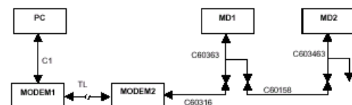
Рис. 4-7 Подключение через телефонную линию: PC: компьютер; MD1, MD2: металлодетекторы; c1: модемный кабель; TL: телефонная линия
