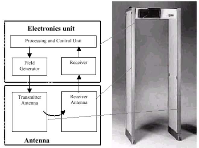
Рис. 1 Блок-схема металлодетектора
